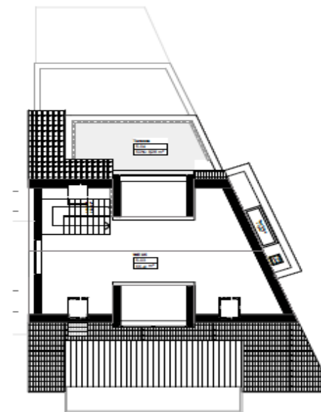
GRUNDRISS Spitzboden
